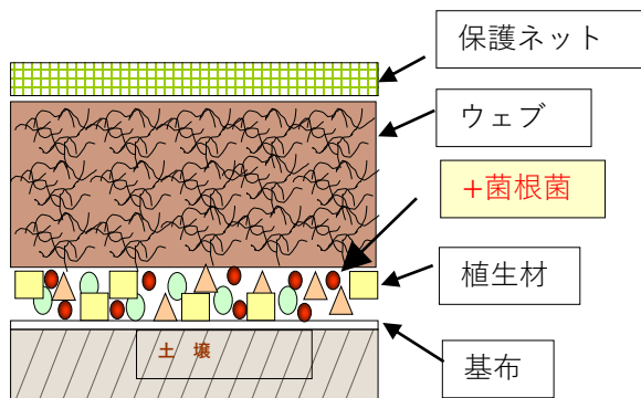
多機能フィルターの基本構造
