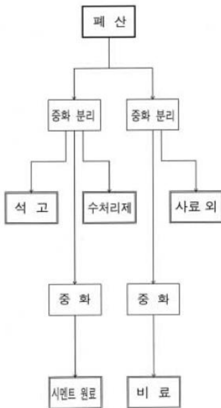
폐산자원화 공정도
