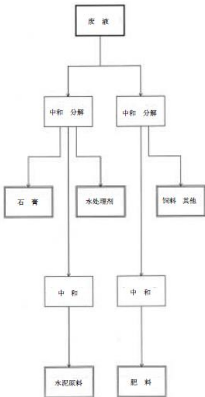
废酸资源化工序图
