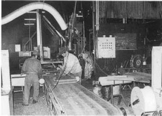
성형연료 제조설비
